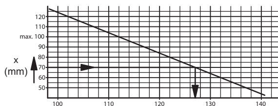
úhel otevření dveří příklad: X = 80 mm ±124° úhel otevření dveří
