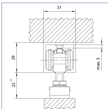
Upevnění do stropu
