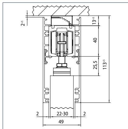
Zacvakávací kryt upevnění do stropu, dřevěné křídlo 22 - 30 mm
