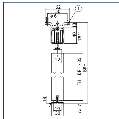
Upevnění do stropu pomocí desky
