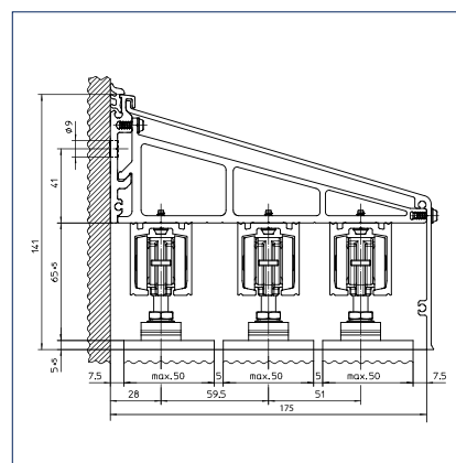
Dlouhá varianta příklad 3-kříd. l.
