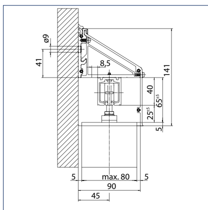
Krátká varianta příklad 1-kříd. l.
