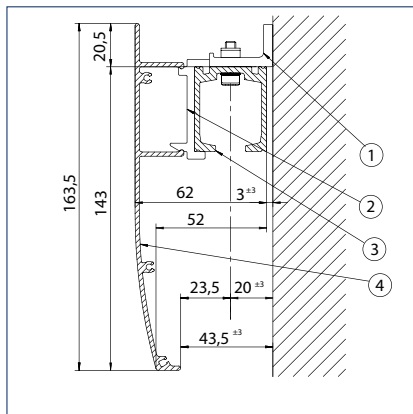
Zacvakávací kryt pro montáž do stěny
