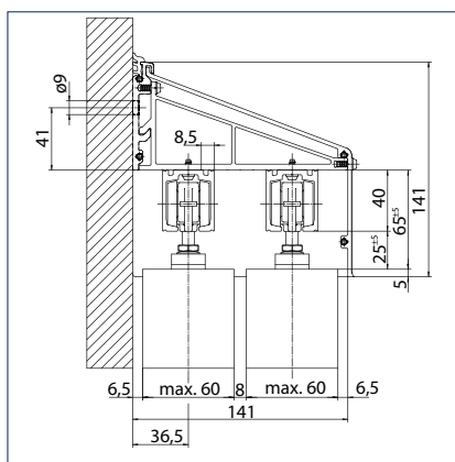
Střední varianta příklad 2-kříd. l.
