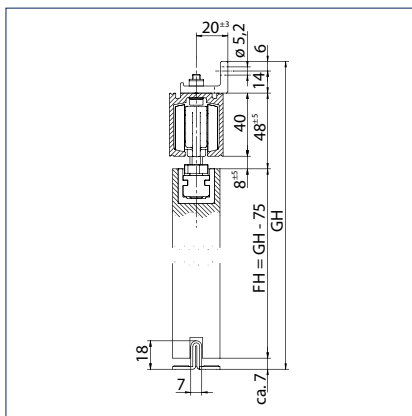
Upevnění do stěny pomocí úhelníku
