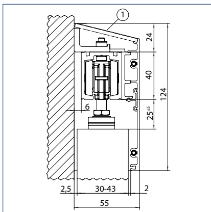
Zacvakávací kryt upevnění do stěny, dřevěné křídlo 30 - 43 mm
