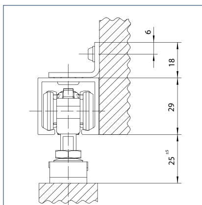
Upevnění do stěny
