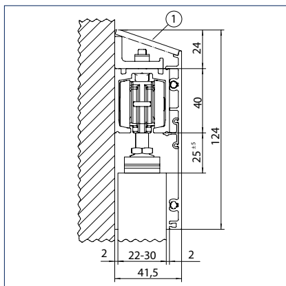
Zacvakávací kryt upevnění do stěny, dřevěné křídlo 22 - 30 mm
