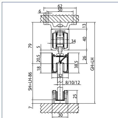
Upevnění do stropu pomocí úhelníku
