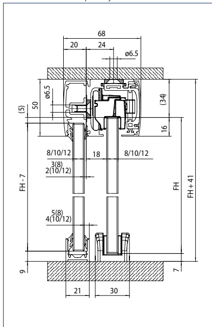
Skleněné křídlo s pevným dílem
