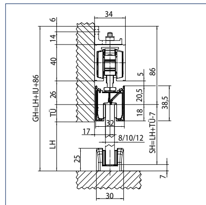
Upevnění na stěnu s GKP 30 mm
