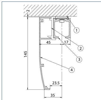
Zacvakávací kryt pro montáž do stropu
