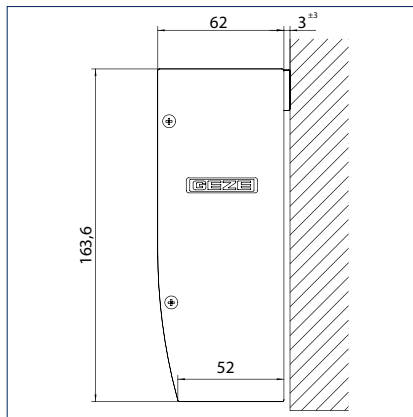
Boční kryt pro montáž do stěny
