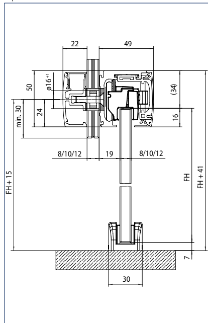
Upevnění na sklo
