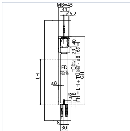
Přímé upevnění do stropu
