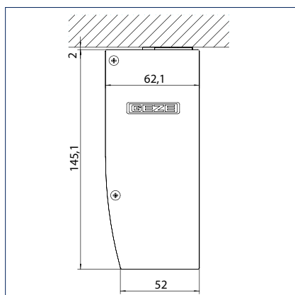
Boční kryt pro montáž do stropu
